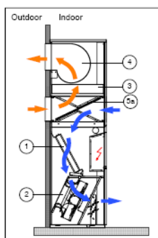
Drift kompressorkøling
