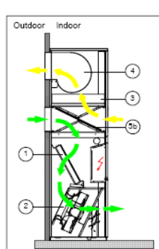
Frikøling udeluft
